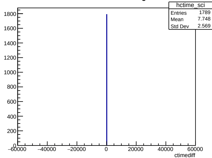
20170208 cosmic scictime-trigtime BF0
